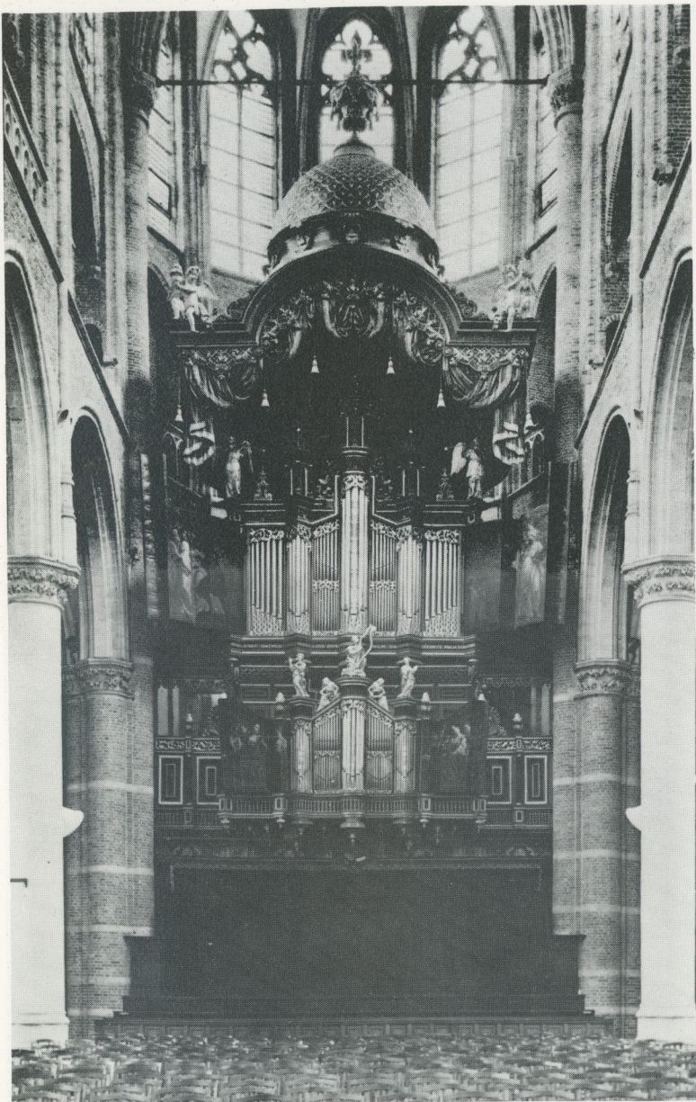
Goes (Zld.), Grote- of Maria Magdalenakerk. Het instrument is vervaardigd door Marcussen, Denemarken in 1970 met gebruikmaking van pijpwerk uit 1710. Kas is uit 1643. Beroemde Turkse kap 1732. Het orgel heeft 39 stemmen, 3 manualen en pedaal.
